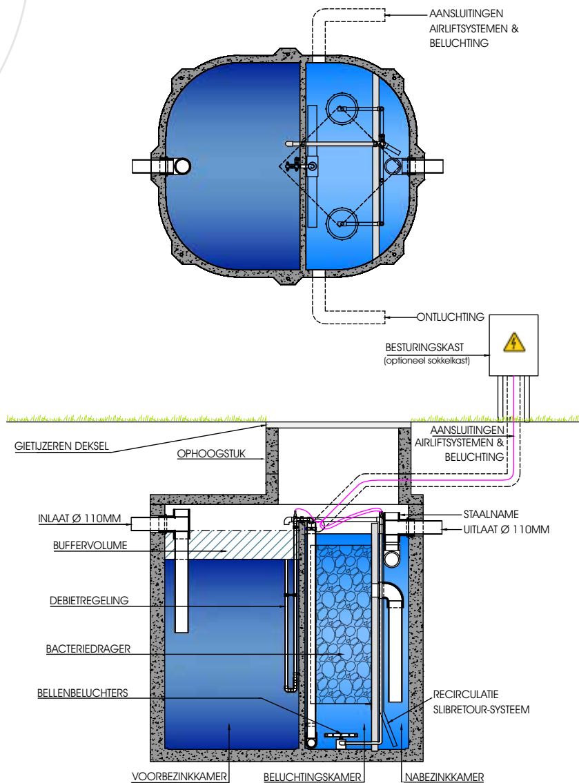
VOORBEELD TYPE BELLEAQUA SAF 1-6 IE
